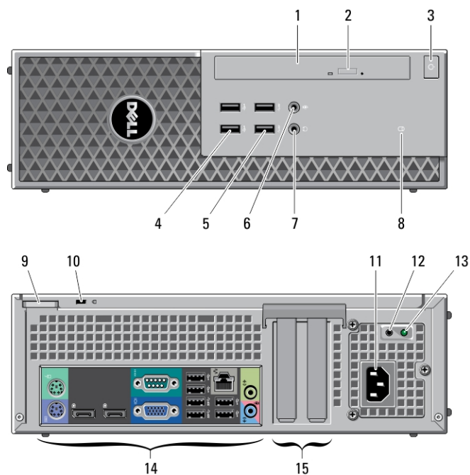
Figura 3. Vistas frontal e traseira do fator de forma pequeno
